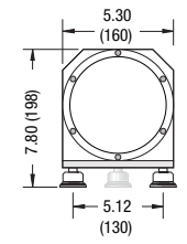
Matisse DS and TS Reference Cell
