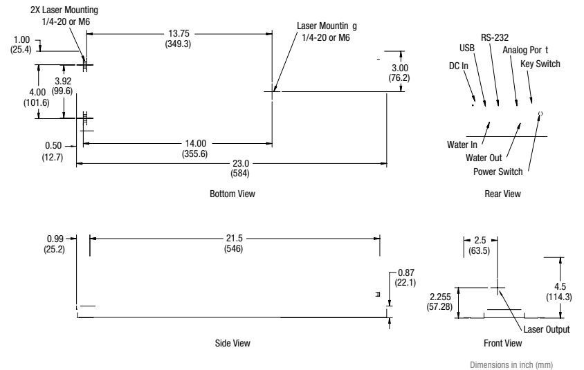
Millennia eV (20-25 W) Dimensions
